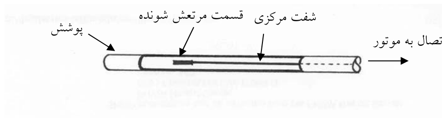
شکل ۳ جزئیات لرزاننده خرطومی
