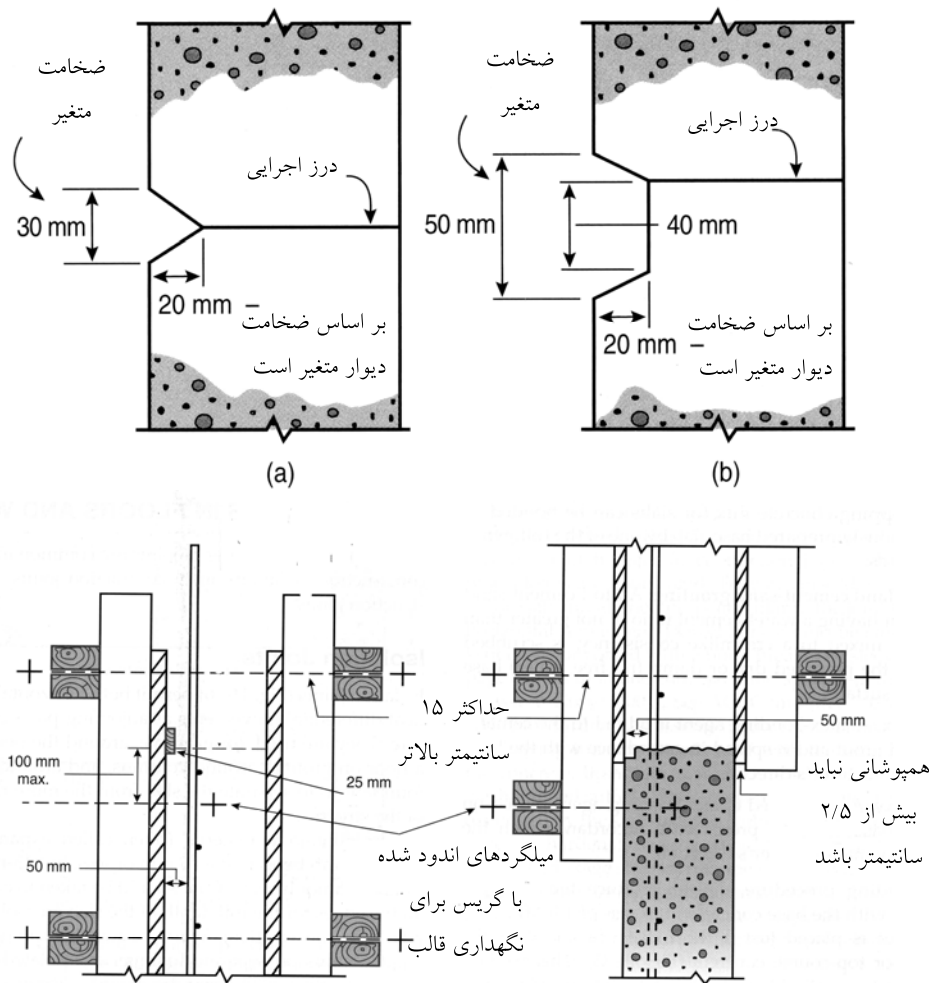
شکل ۱ درز ساخت
